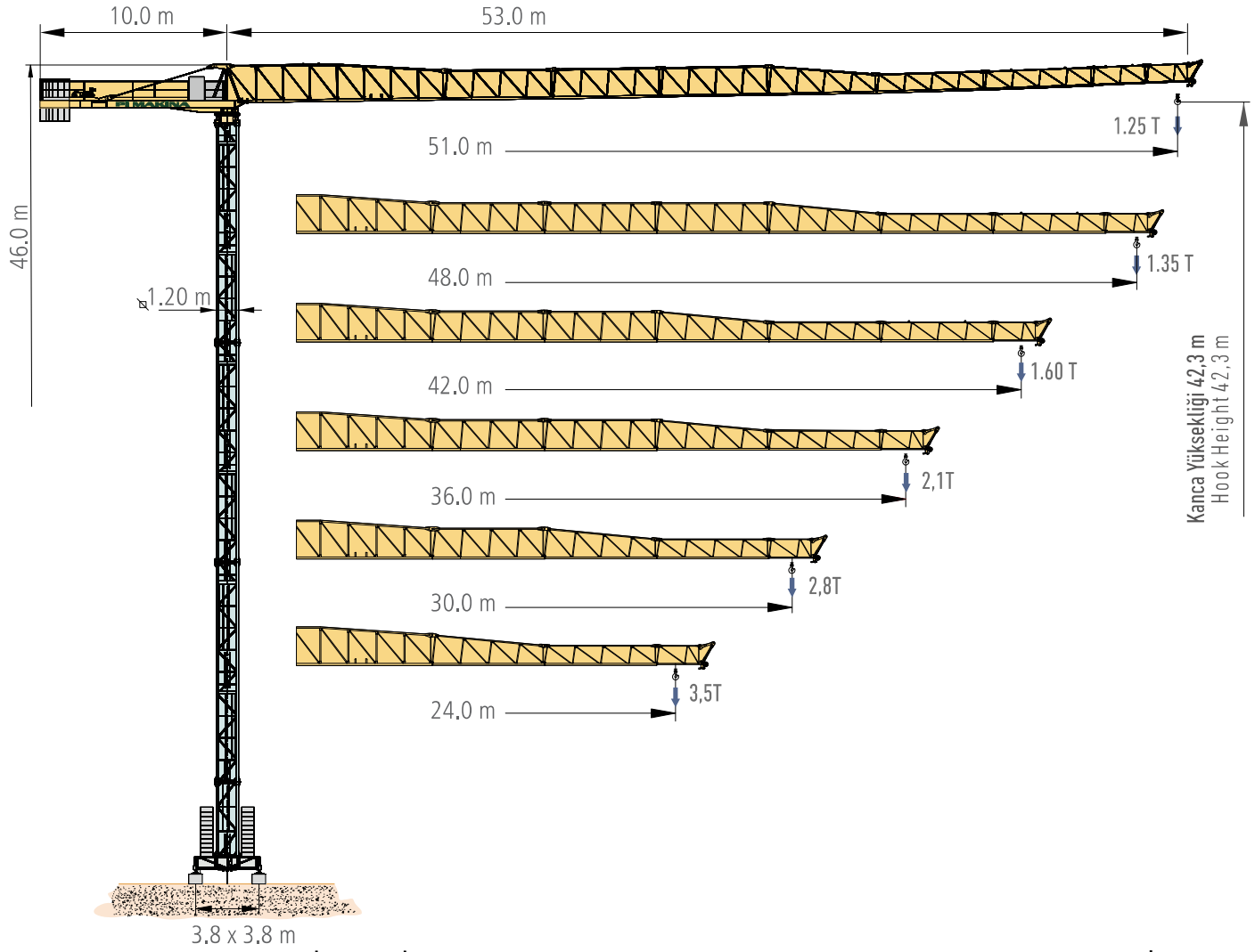
SABİT TABLA
